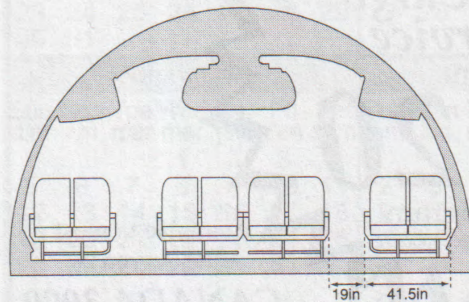
Wide Bodied Twin Aisle with 4 Double Seats Gros porteur, deux allées avec 4 sièges doubles
